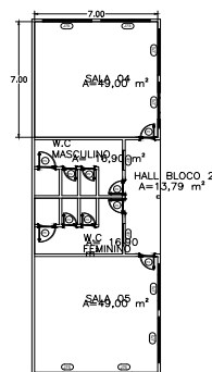
01 PLANTA BAIXA - BLOCO I
